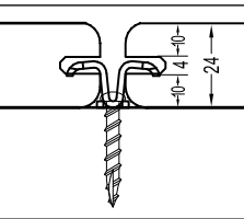
Schéma de fixation COBRA® 24
