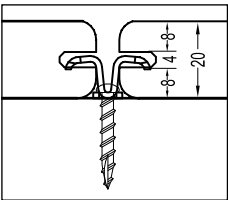
Schéma de fixation COBRA® 20
